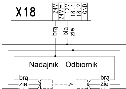
Rayector bramka świetlna lub listwa optyczna jako zabezpieczenie przed wciągnięciem pojedyncza
