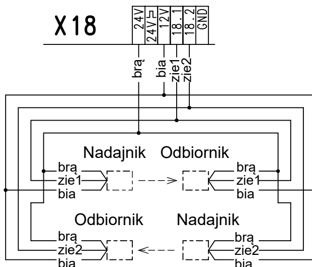
Rayector bramka świetlna lub listwa optyczna jako zabezpieczenie przed wciągnięciem podwójna
